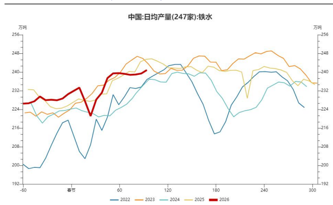
图 14：日均铁水产量上升
